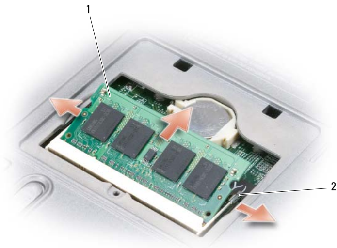
1 記憶體模組
